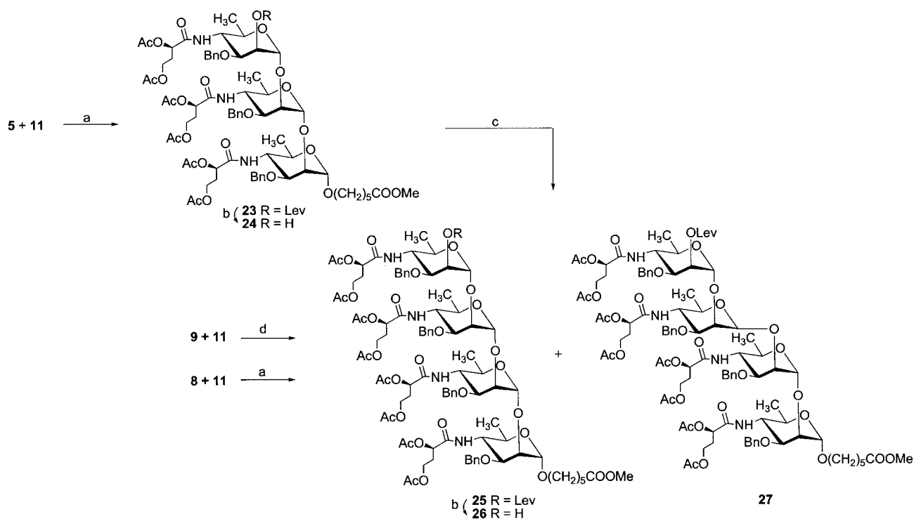
Scheme 3. a: NIS, AgOTf, CH 2 Cl 2 ; b: H 2 NNH 2 ·AcOH, CH 2 Cl 2 /MeOH; c: 5 , NIS, AgOTf, CH 2 Cl 2 ; d: AgOTf, 2,6-di- tert -butyl-4-methylpyridine, CH 2 Cl 2 .
